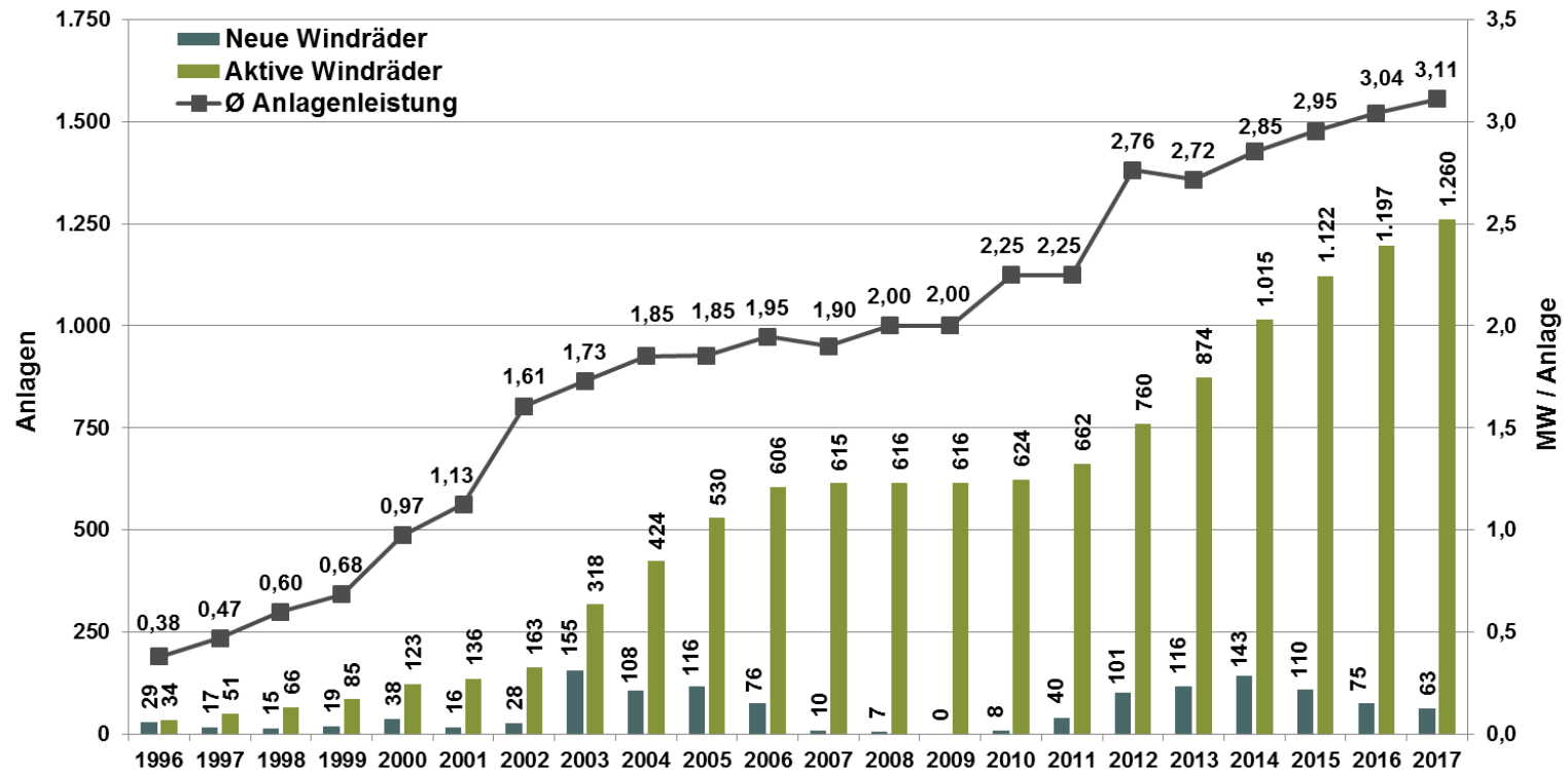
Abbildung 2: Jährlicher Neubau von Windrädern, Anzahl aller aktiven Windräder und durchschnittliche Anlagenleistung von WKA
