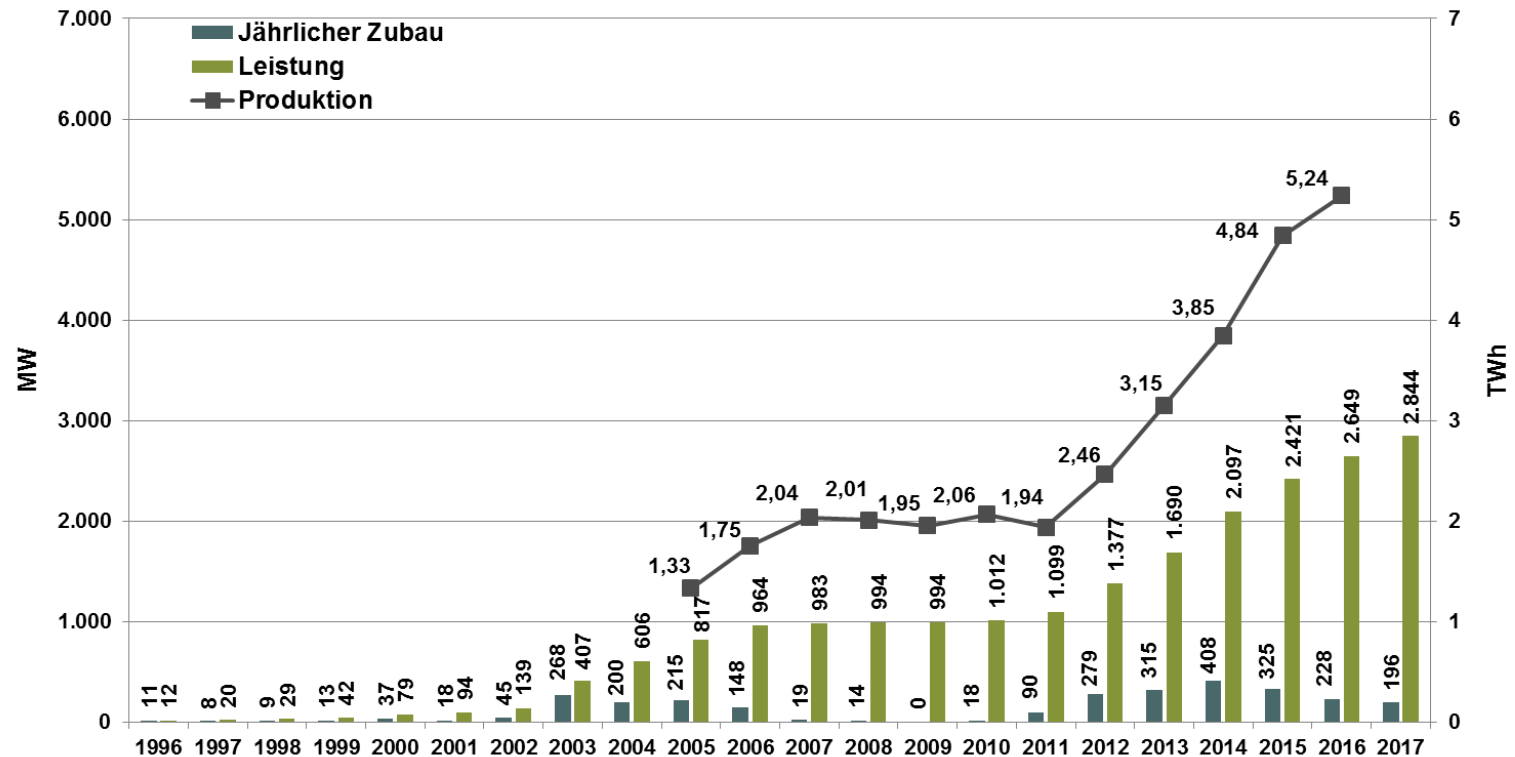
Abbildung 1: Jährlicher Zubau (in MW), Gesamtleistung (in MW) und –produktion (TWh) von Strom durch Windkraft in Österreich
